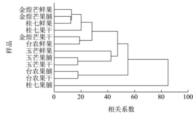
图 6 不同品种芒果鲜果、果脯及果干的聚类分析
