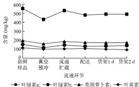
图 11 5.0 °C 流通温度下流通环节苏州青叶片叶绿素 a、叶绿素 b、叶黄素和类胡萝卜素含量的变化
